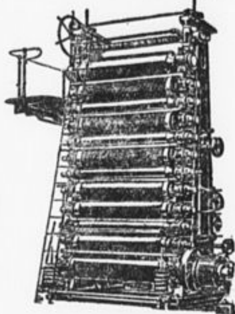
Каландр в шлифовальной машине.
